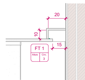
2 CORTE - FORRO ESCALA: 1 : 25
