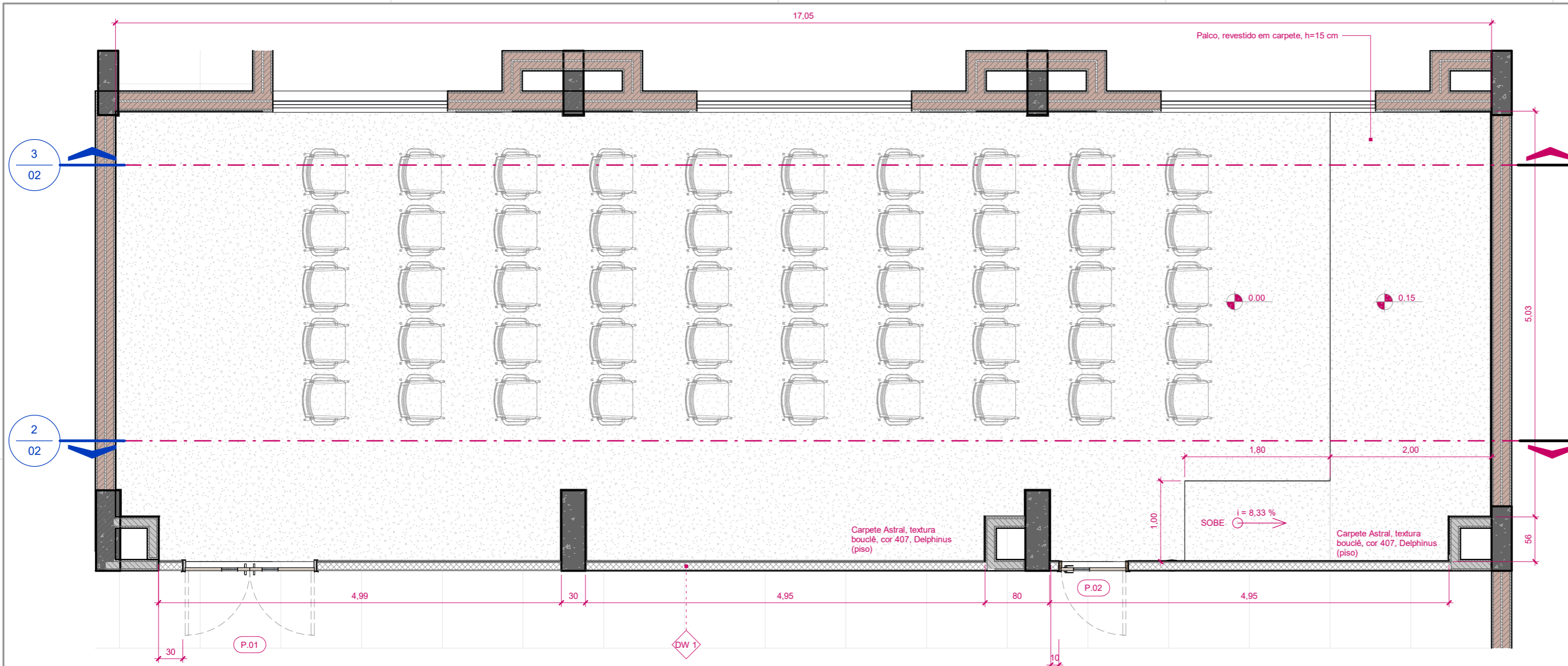
1 Superior(2) ESCALA: 1 : 50
