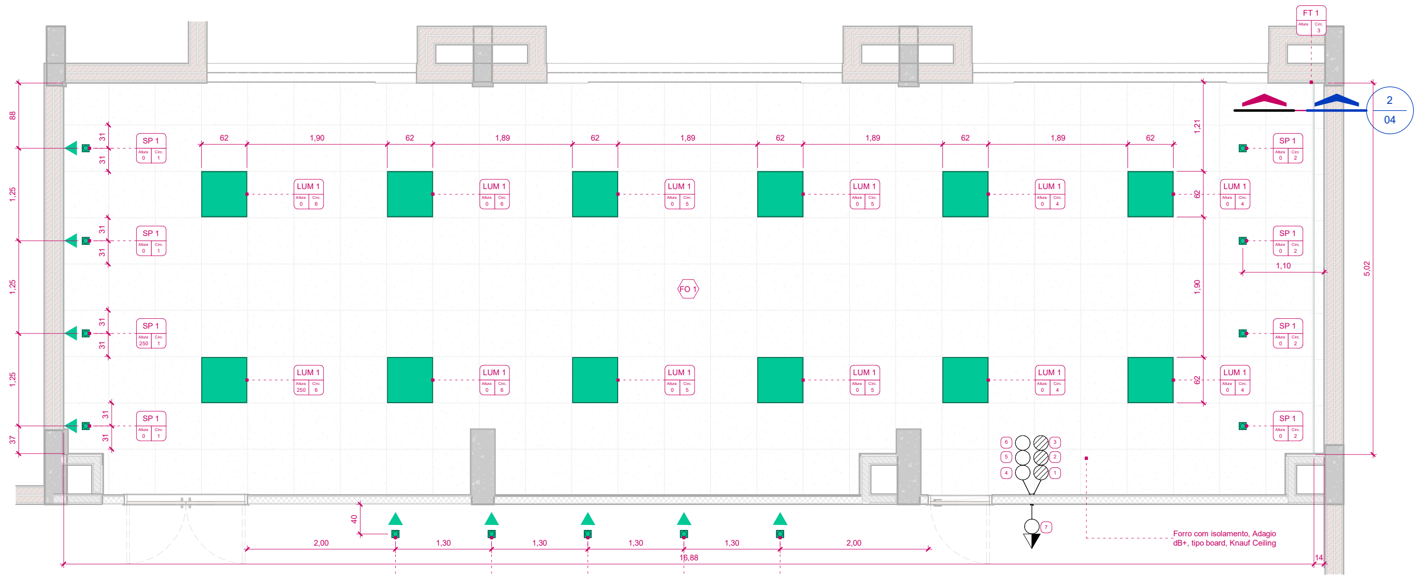
1 PLANTA DE FORRO - LUMINOTÉCNICO ESCALA: 1 : 50
