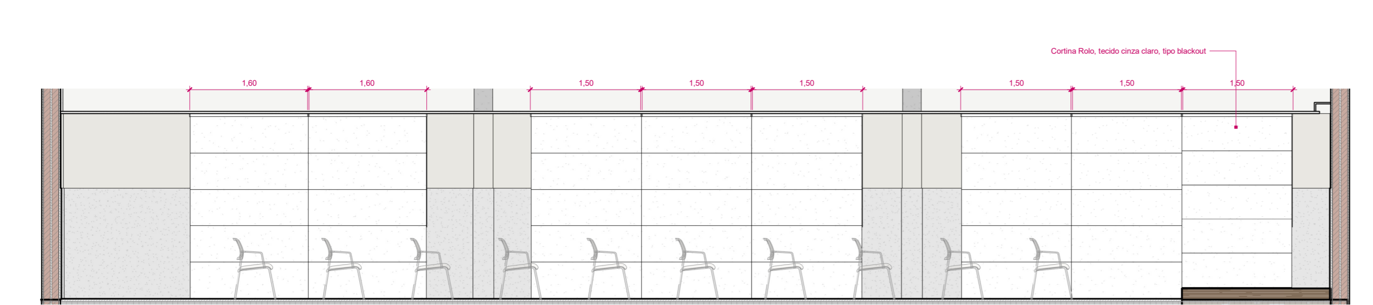
3 Section 3 ESCALA: 1 : 50
