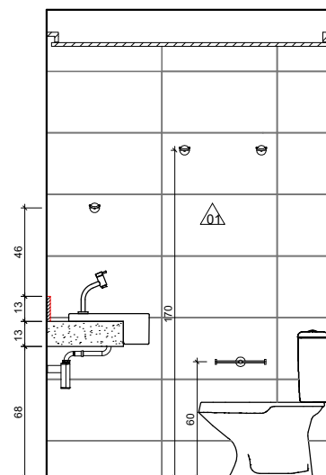
VISTA A ESCALA 1/25
