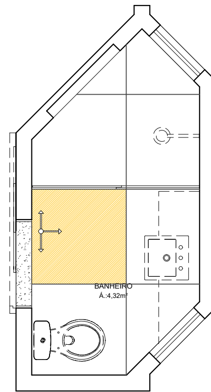
PAGINAÇÃO DE PISO ESCALA 1/25
