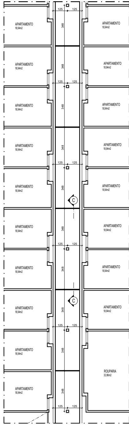
PLANTA TETO REBATIDO 1º PAVIMENTO TRECHO 02 ESCALA 1/125
