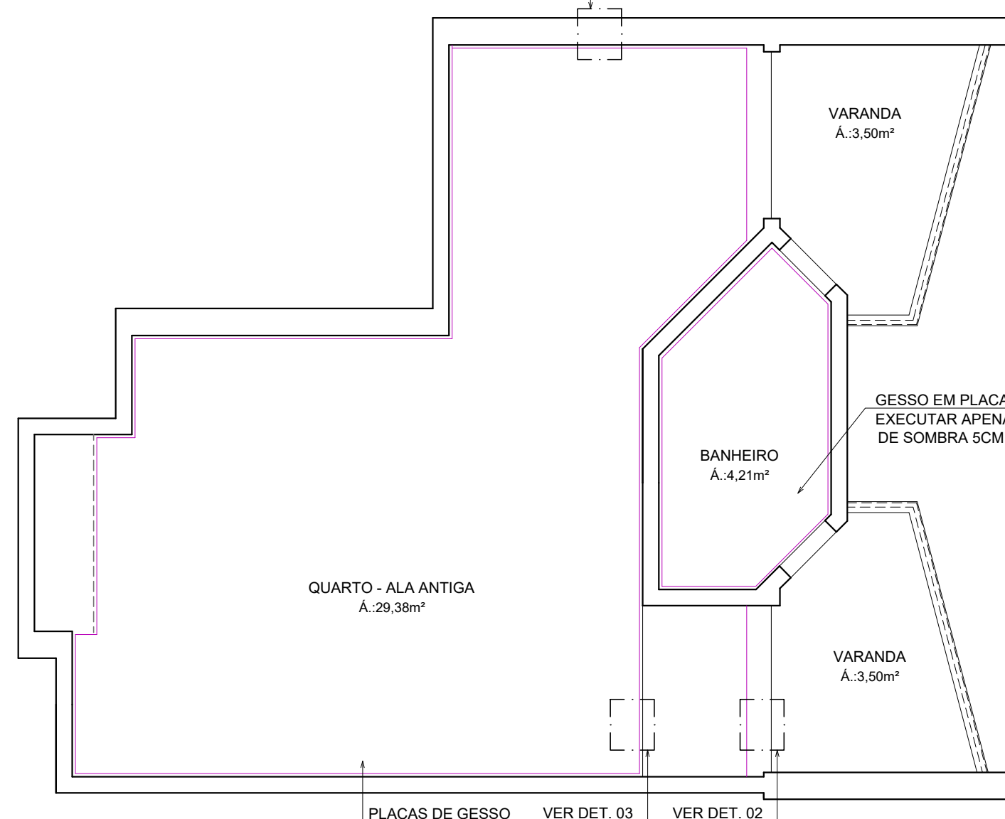
PLANTA TETO REBATIDO TÉRREO / 1º PAV ESCALA 1/50
