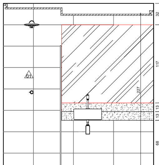
VISTA B ESCALA 1/25
