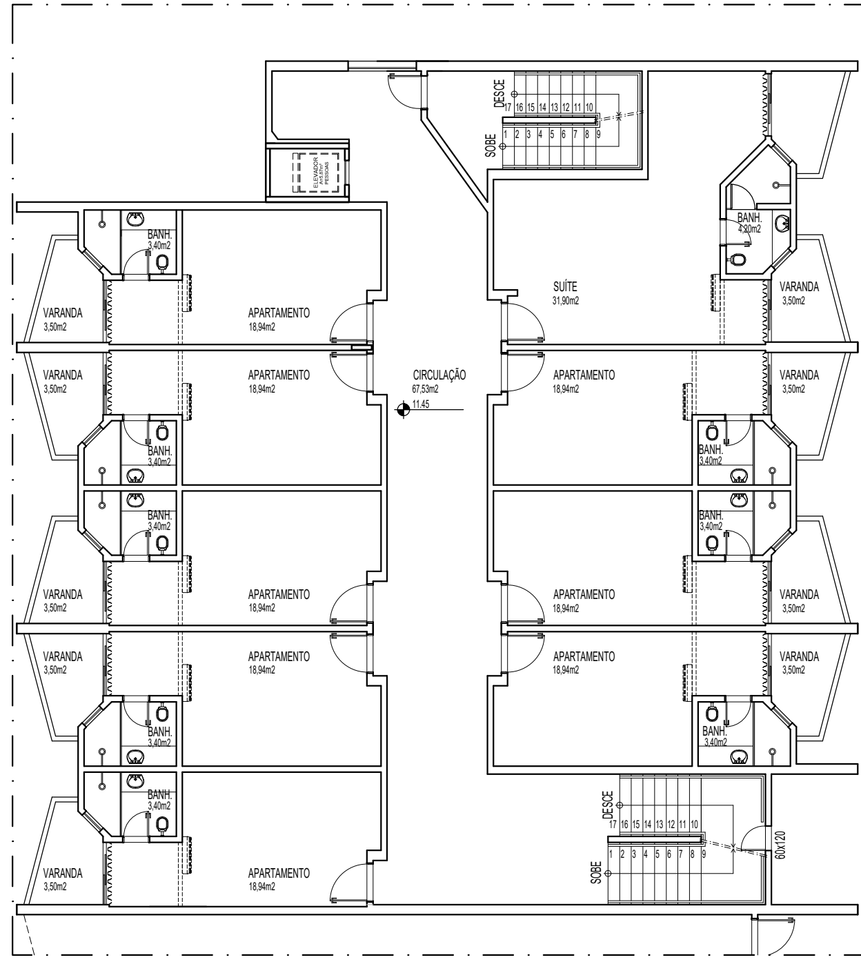
PLANTA BAIXA 1º SUBSOLO EXISTENTE ESCALA 1/125 APTOS 352 A 359
