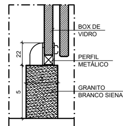
DETALHE BOX SEM ESCALA
