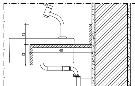
DET. BANCADA ESCALA 1/10
