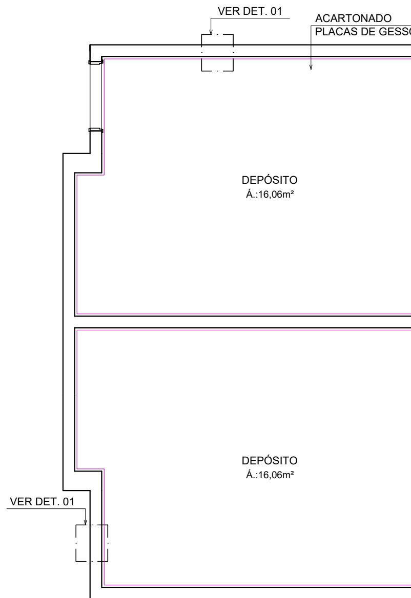
PLANTA TETO REBATIDO ESCALA 1/50
