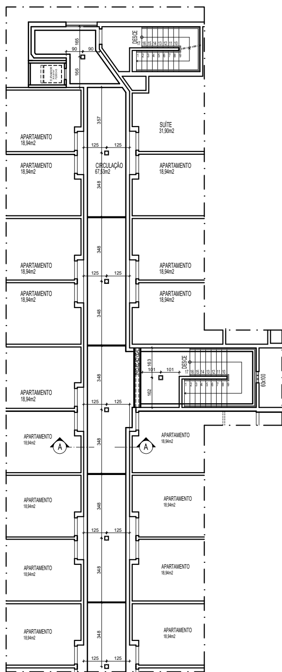
PLANTA TETO REBATIDO 1º PAVIMENTO TRECHO 01 ESCALA 1/125
