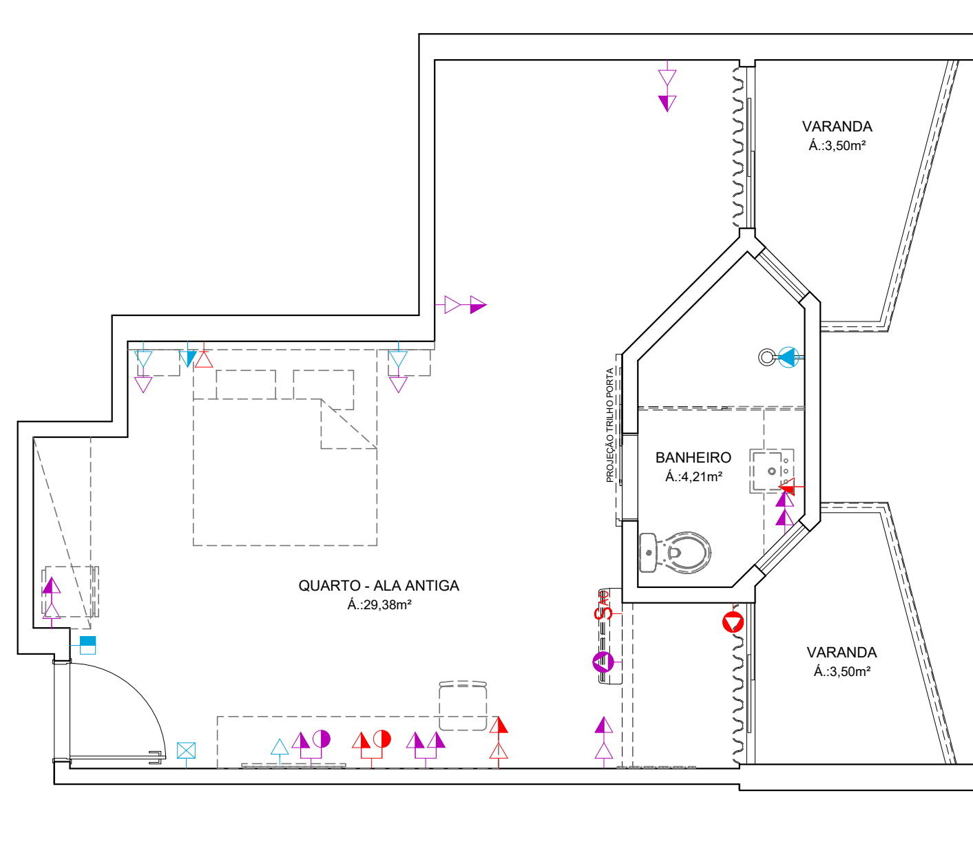
PLANTA BAIXA - PONTOS ELÉTRICOS ESCALA 1/50
