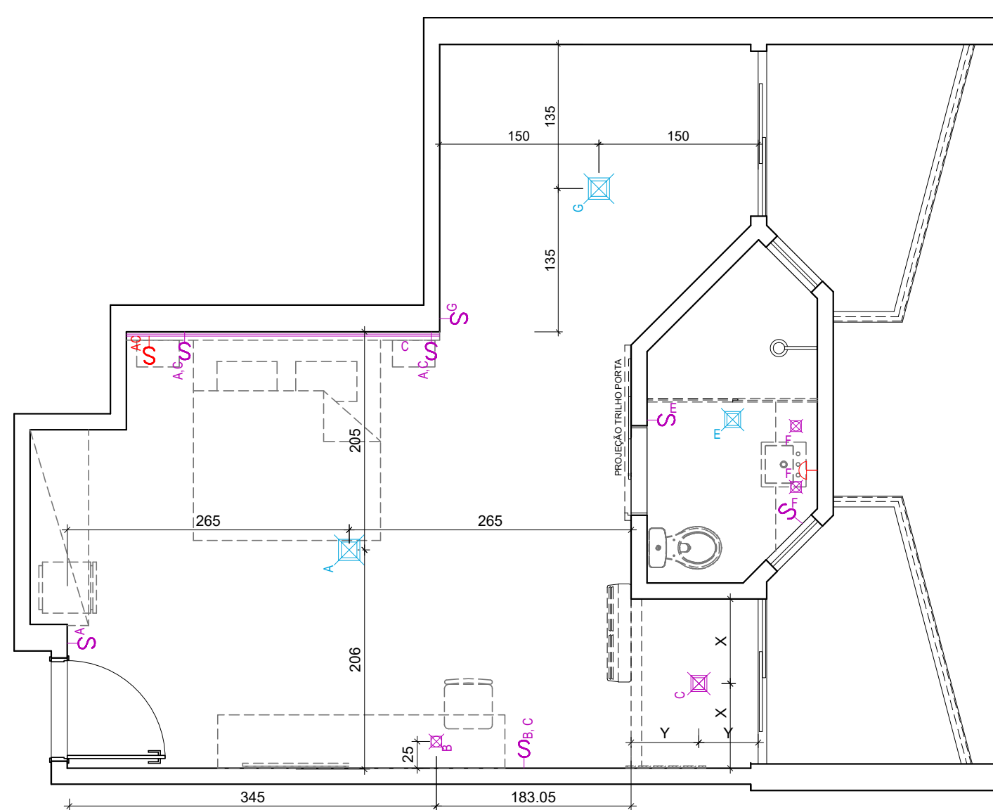
PLANTA BAIXA - ILUMINAÇÃO TÉRREO / 1º PAV ESCALA 1/50
