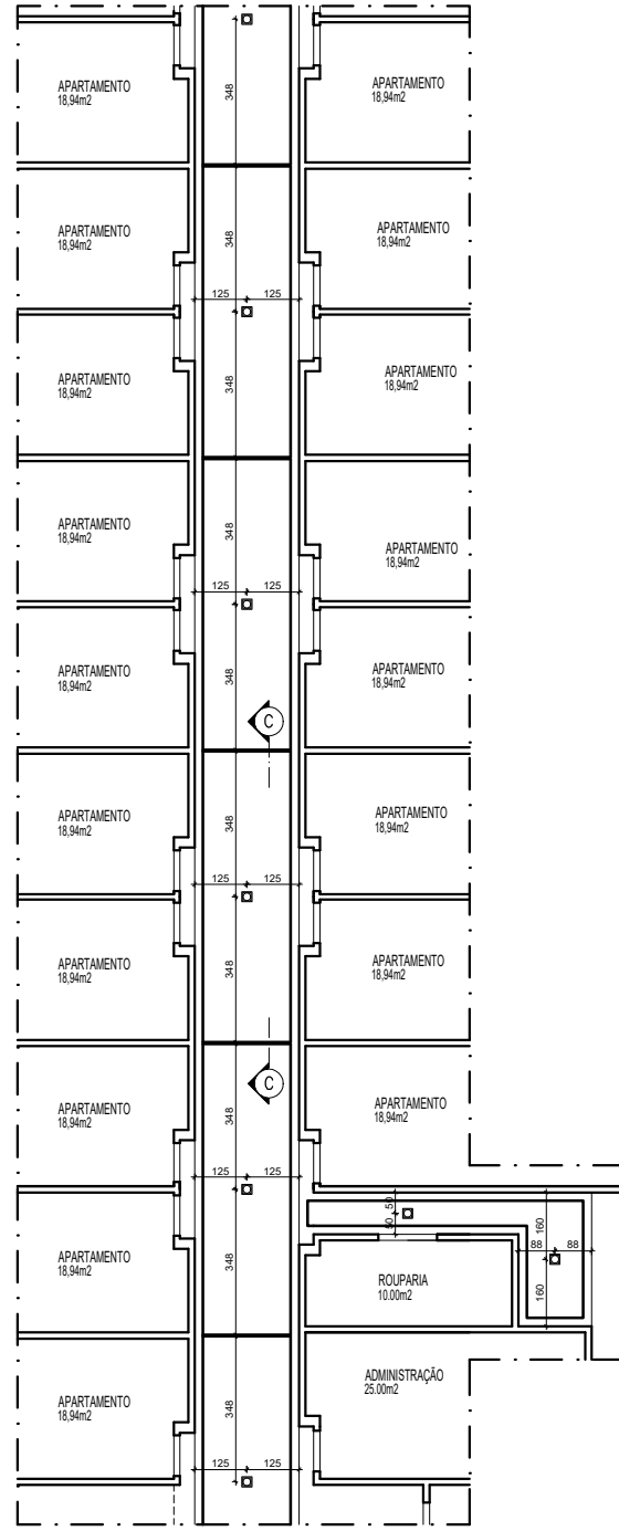
PLANTA TETO REBATIDO TÉRREO TRECHO 02 ESCALA 1/125
