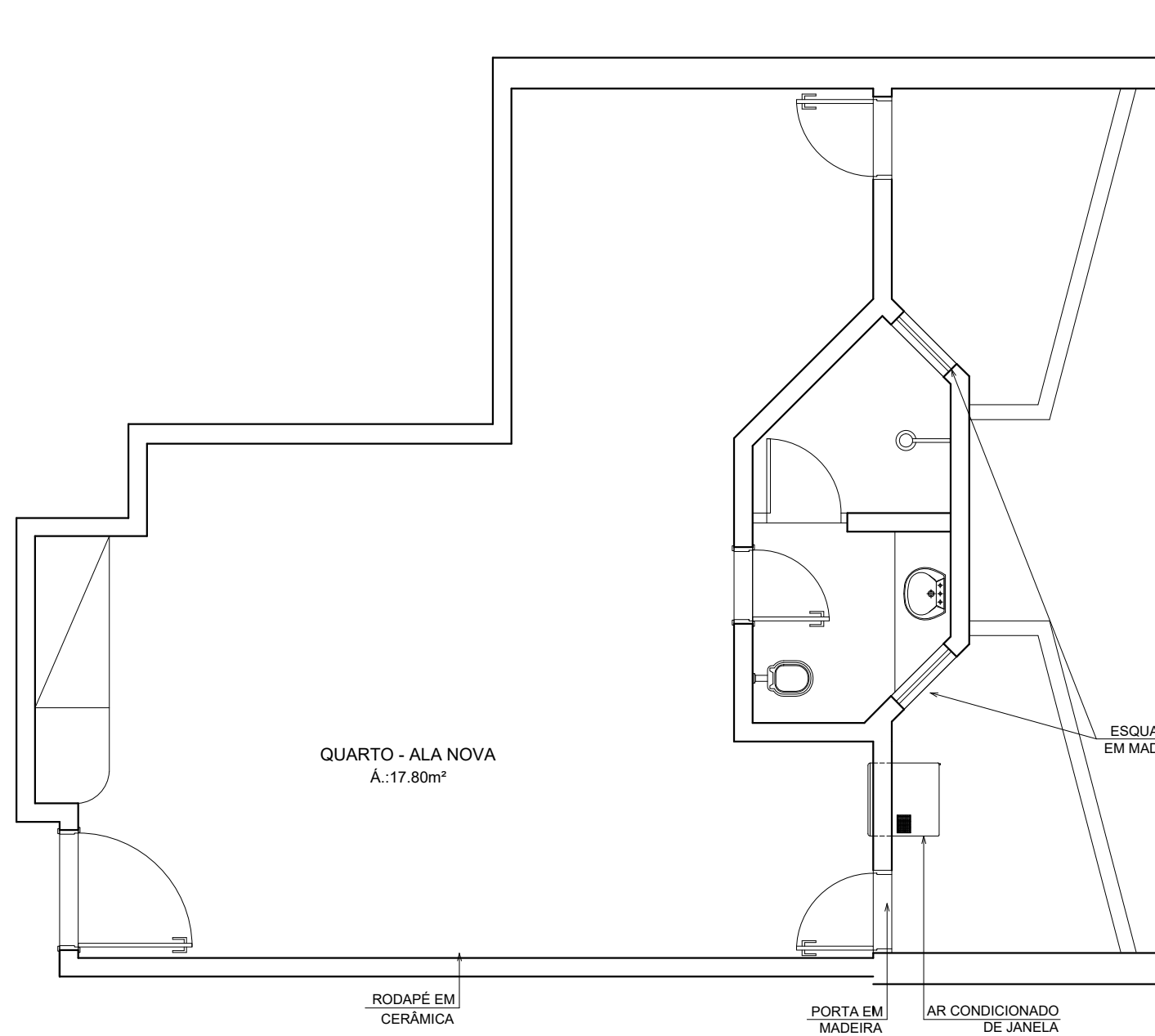
PLANTA BAIXA - ORIGINAL ESCALA 1/50
