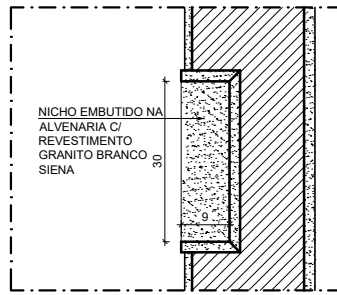
DET. NICHOS ESCALA 1/10
