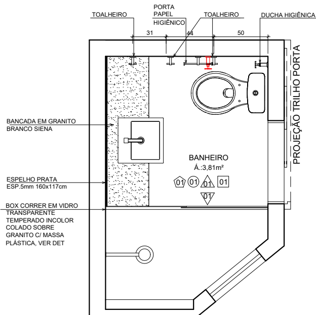
PLANTA LAYOUT ESCALA 1/25
