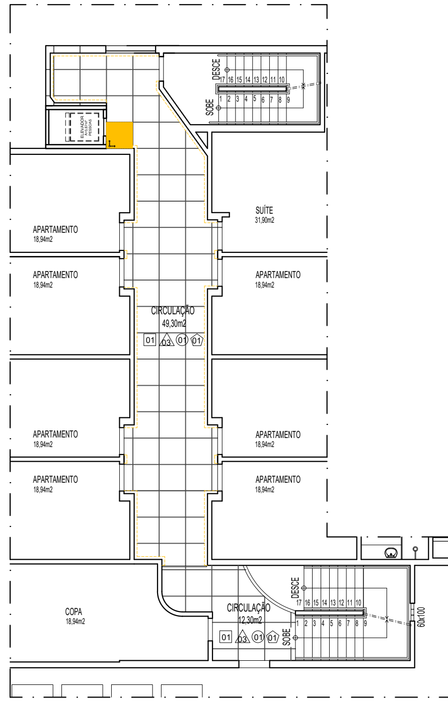
PLANTA PAGINAÇÃO DE PISO SUBSOLO ESCALA 1/125
