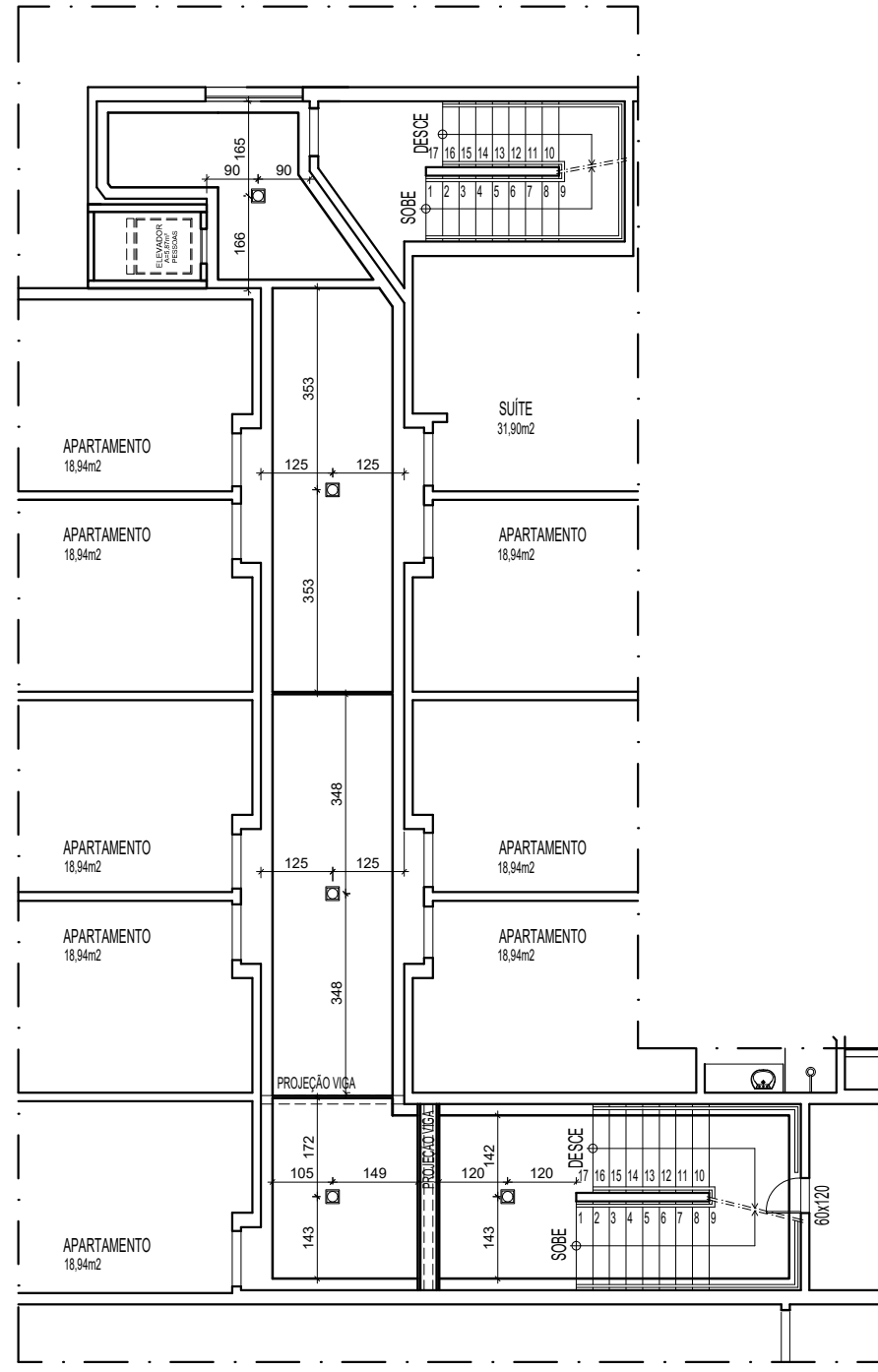
PLANTA TETO REBATIDO 1º SUBSOLO ESCALA 1/125
