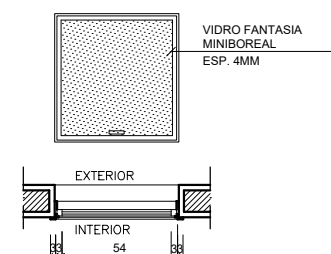
DETALHES JANELA ESCALA 1/10
