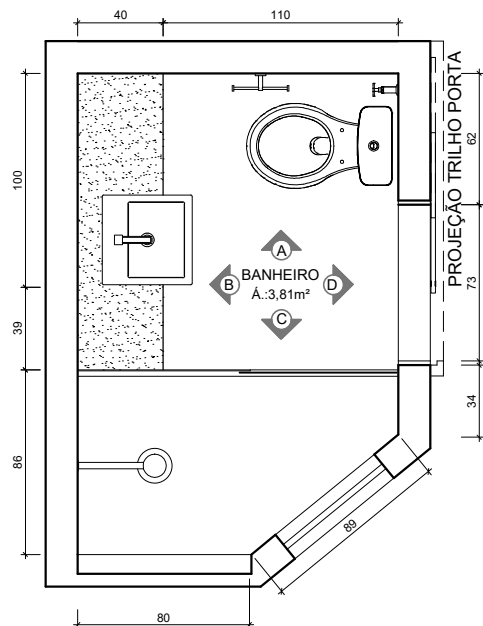
PLANTA BAIXA ESCALA 1/25
