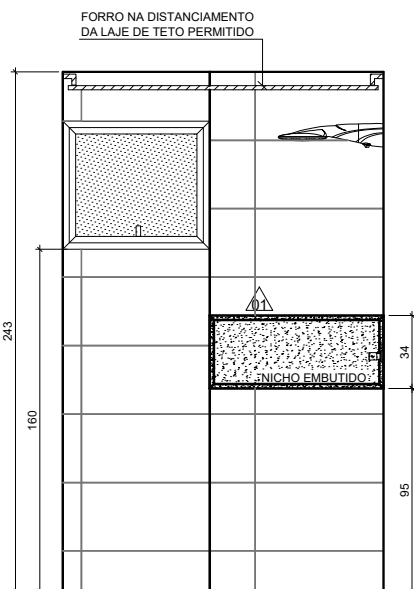
VISTA C ESCALA 1/25
