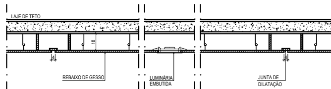
CORTE CC - GESSO ESCALA 1/20
