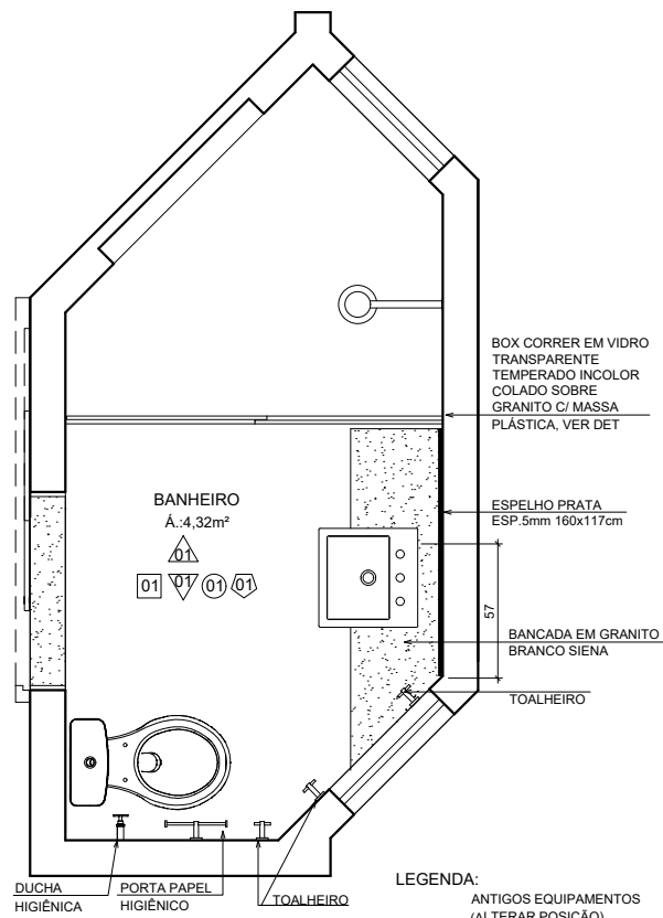
PLANTA LAYOUT ESCALA 1/25
