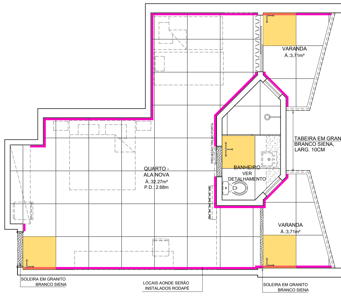
PLANTA PAGINAÇÃO DE PISO ESCALA 1/50
