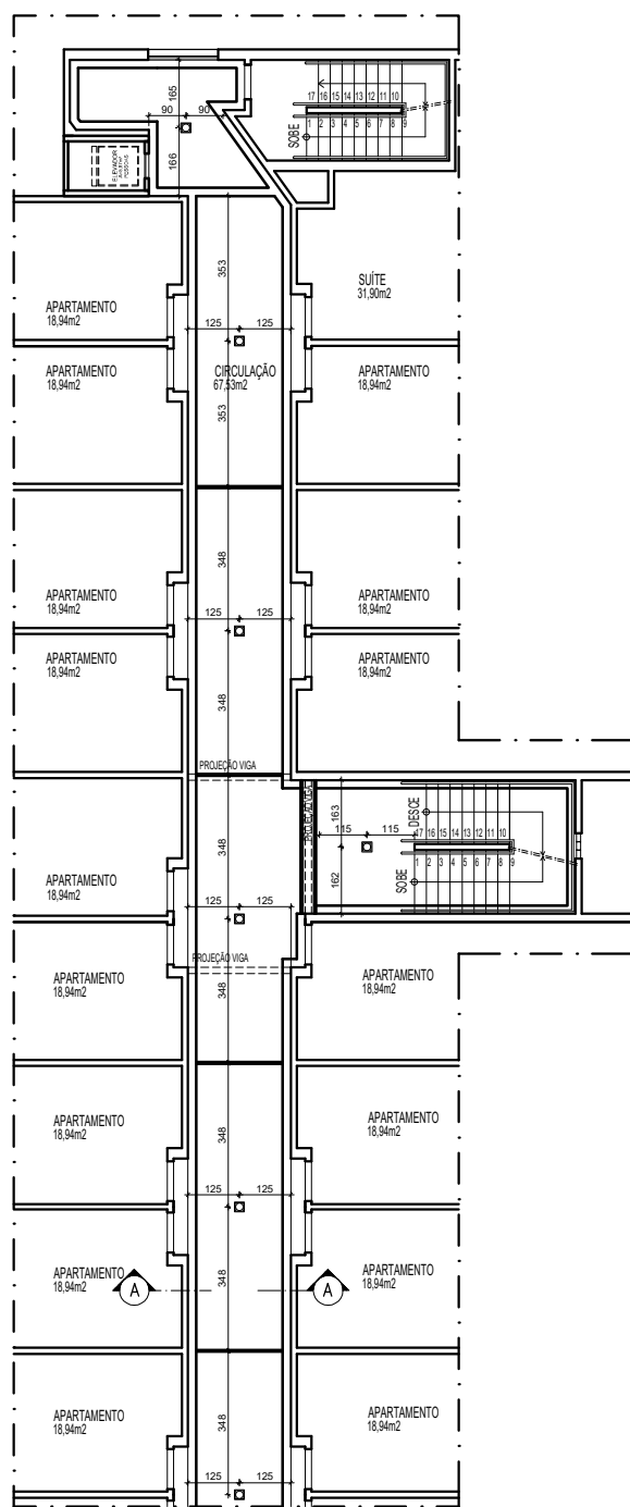
PLANTA TETO REBATIDO TÉRREO TRECHO 01 ESCALA 1/125
