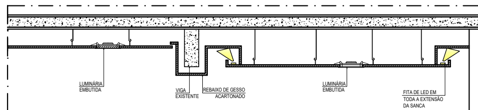
CORTE DD - GESSO ESCALA 1/20
