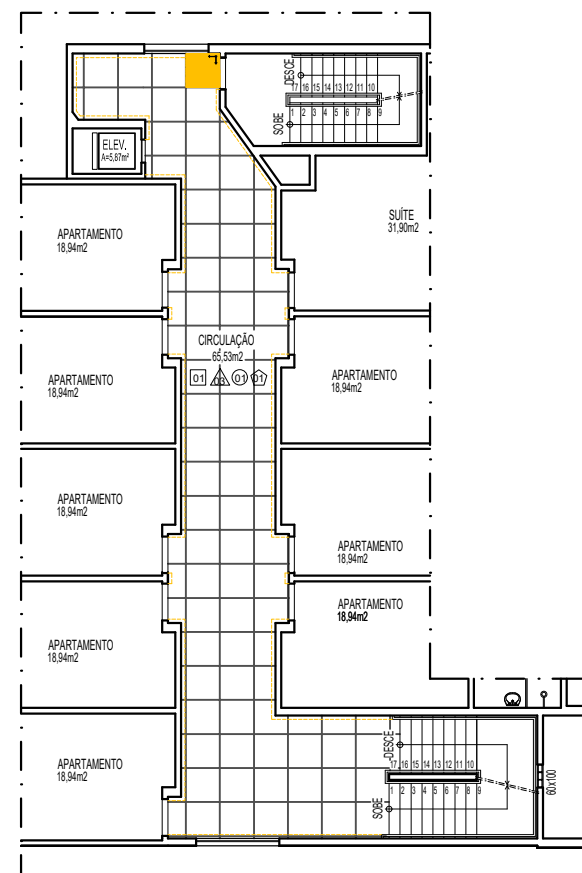
PLANTA PAGINAÇÃO DE PISO 2º E 3º PAVIMENTO ESCALA 1/125
