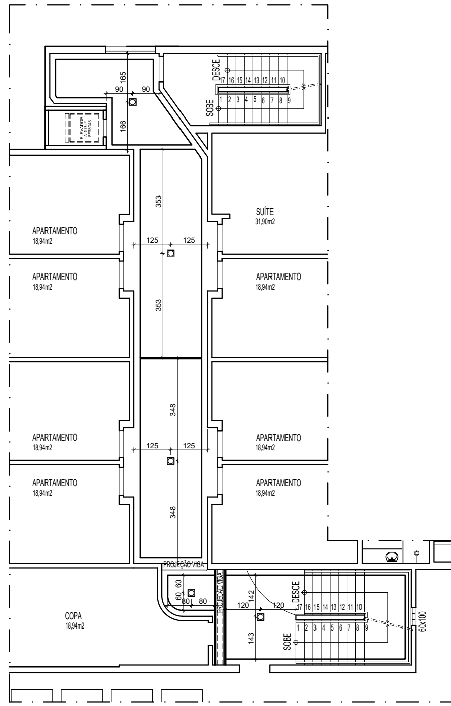
PLANTA TETO REBATIDO SUBSOLO ESCALA 1/125
