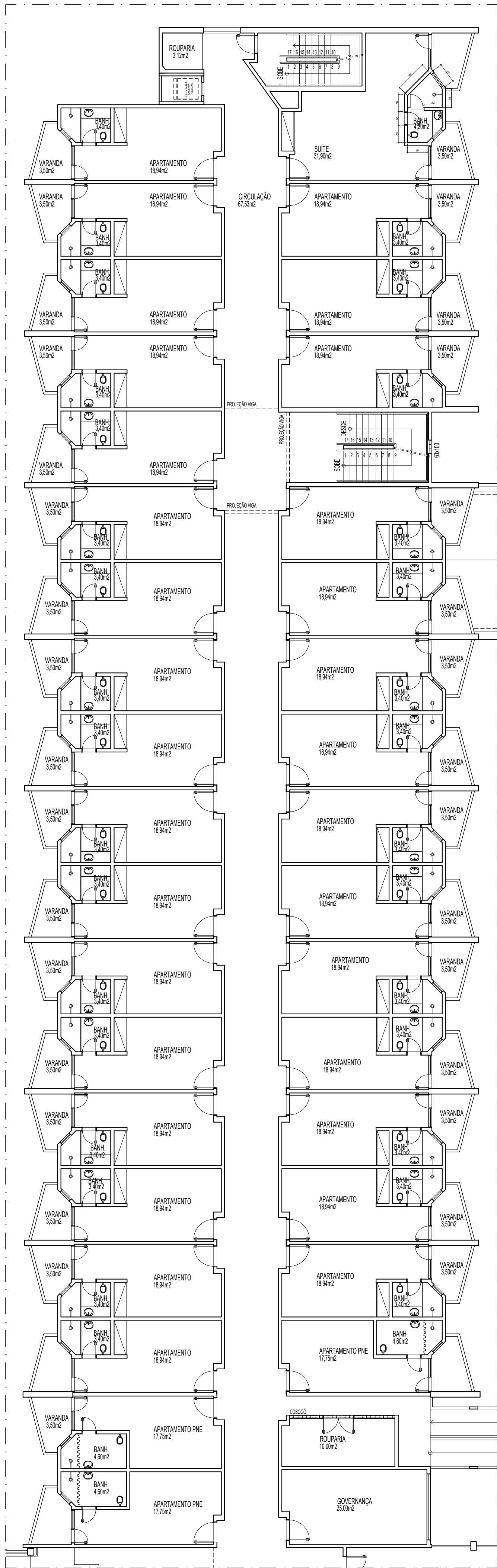
PLANTA BAIXA TÉRREO ESCALA 1/125 APTOS 360 A 394
