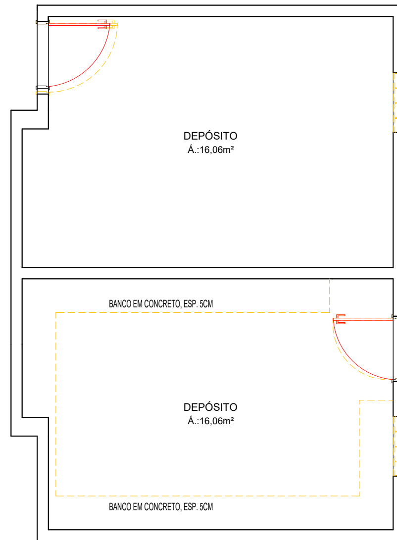
PLANTA BAIXA - DEMOLIÇÃO ESCALA 1/50
