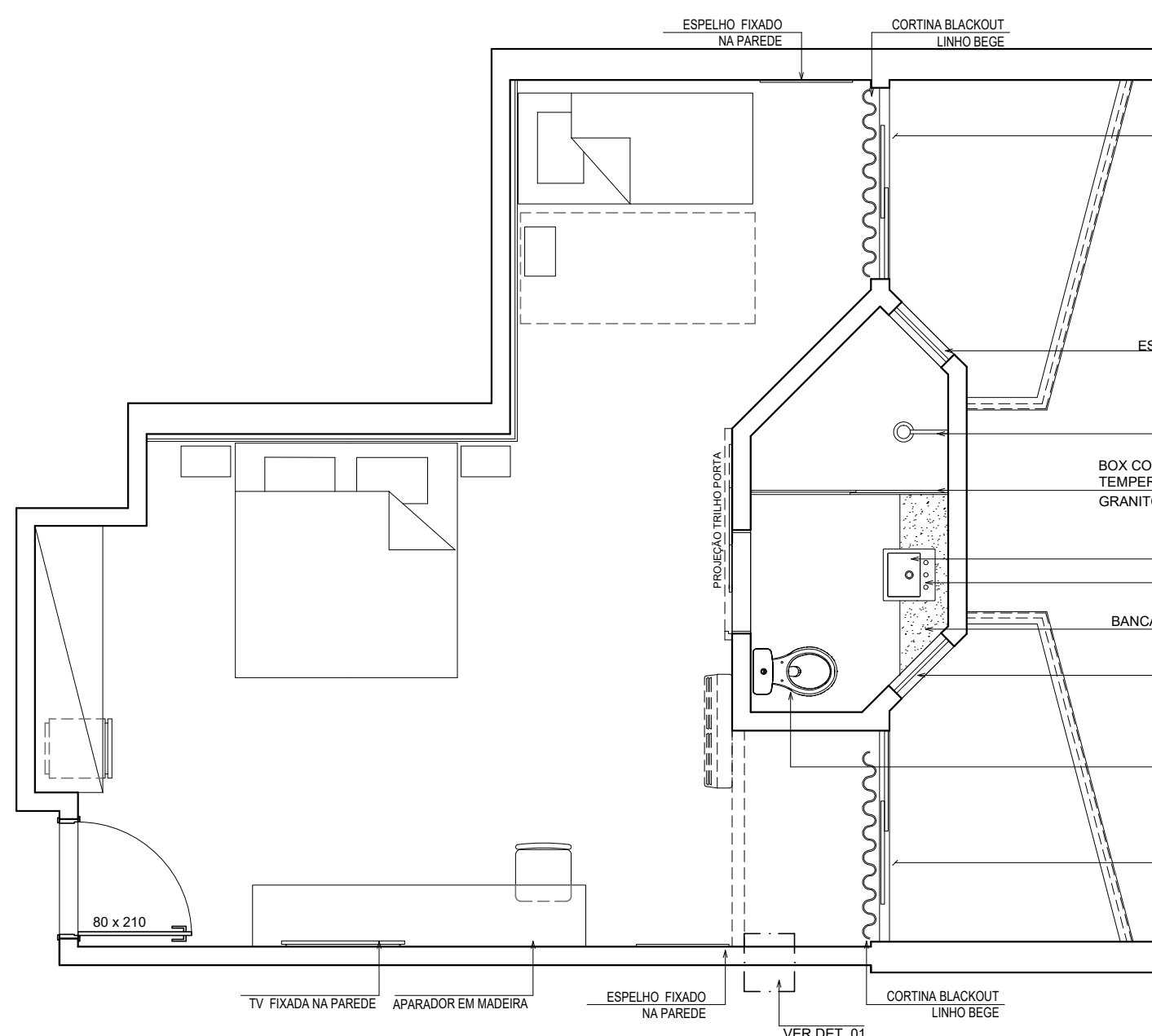
PLANTA BAIXA - LAYOUT ESCALA 1/50
