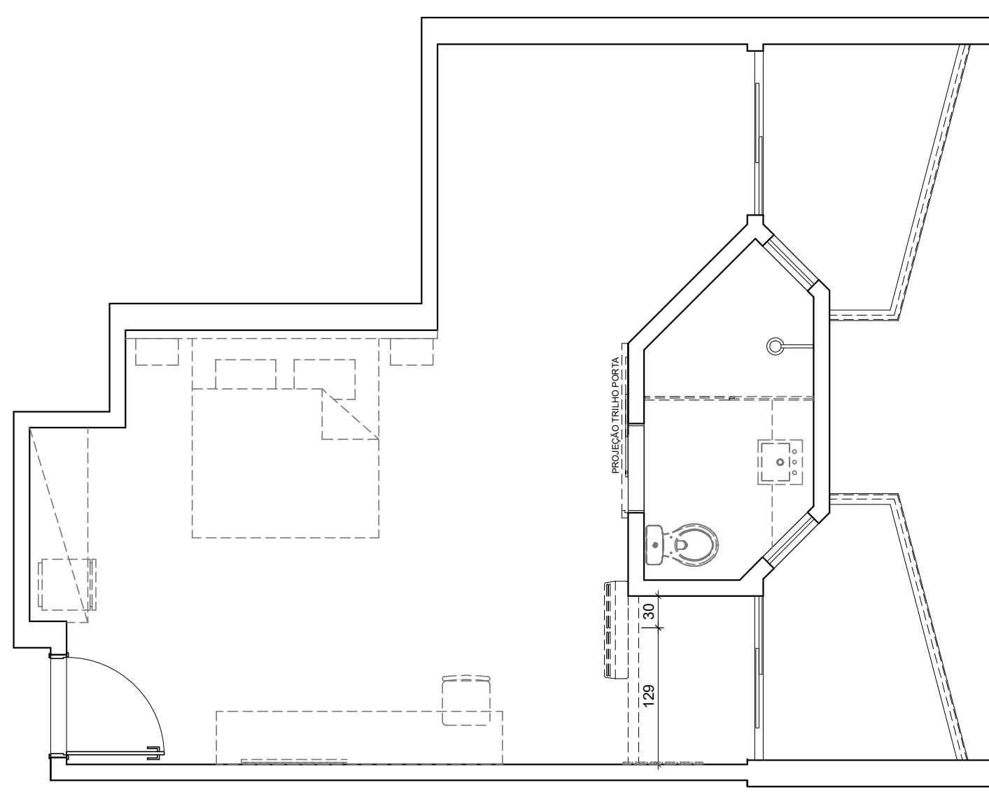
PLANTA BAIXA - AR CONDICIONADO TÉRREO / 1º PAV ESCALA 1/50
