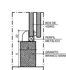
DETALHE BOX SEM ESCALA
