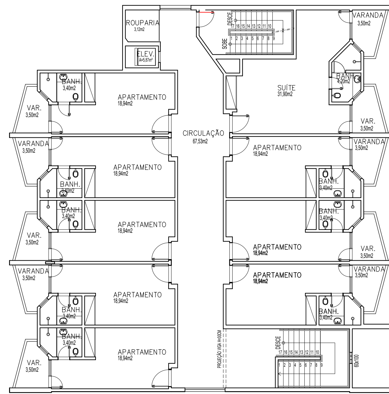
PLANTA BAIXA 3º PAVIMENTO ESCALA 1/125 APTOS 439 A 447
