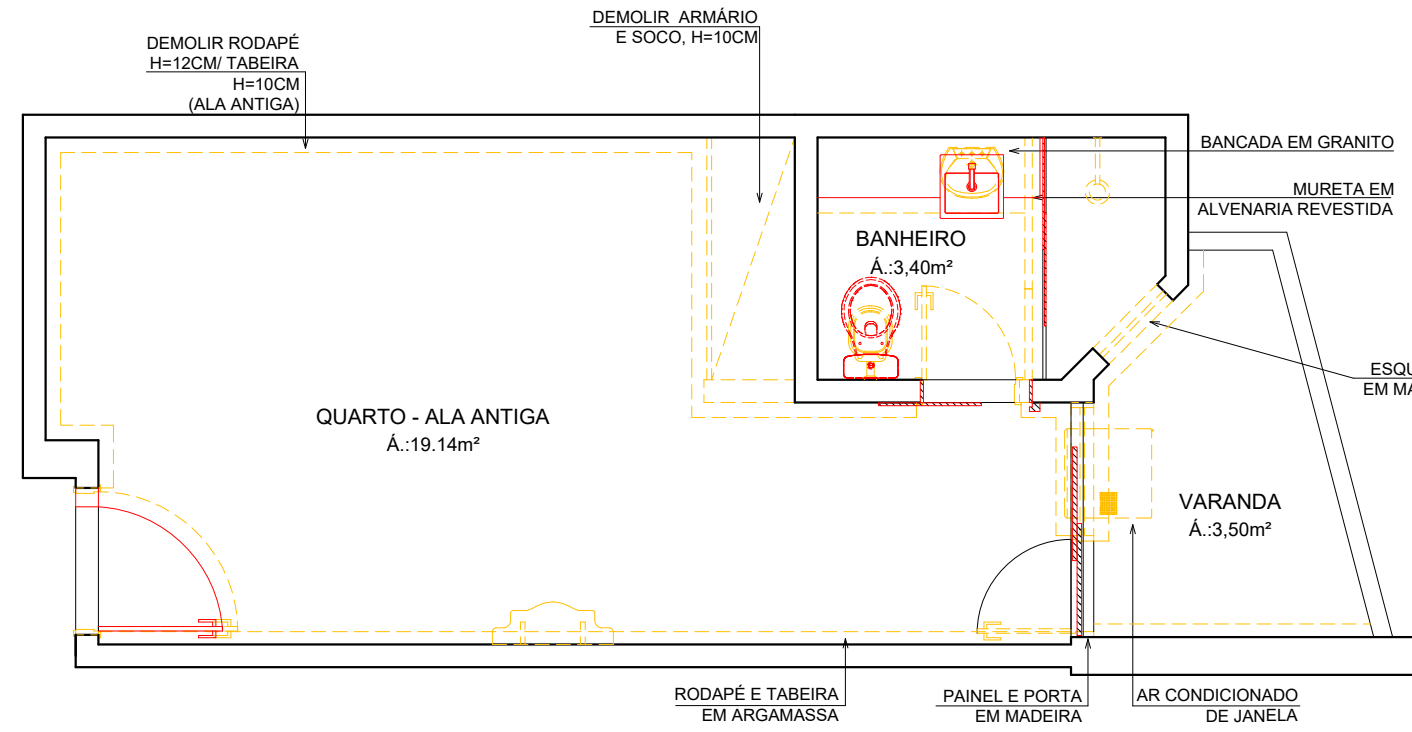
PLANTA BAIXA - DEMOLIÇÃO ESCALA 1/50
