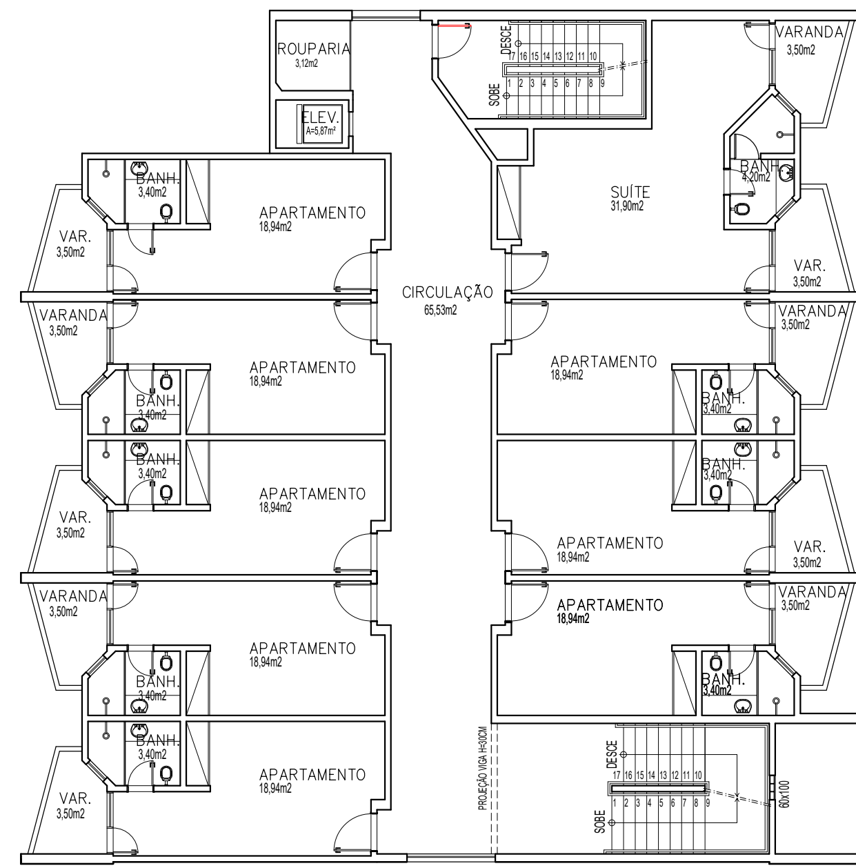
PLANTA BAIXA 2º PAVIMENTO ESCALA 1/125 APTOS 430 A 438
