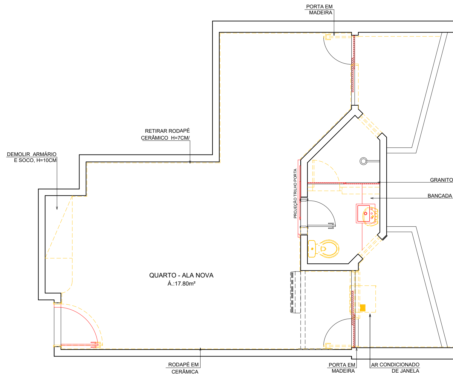
PLANTA BAIXA - DEMOLIÇÃO ESCALA 1/50
