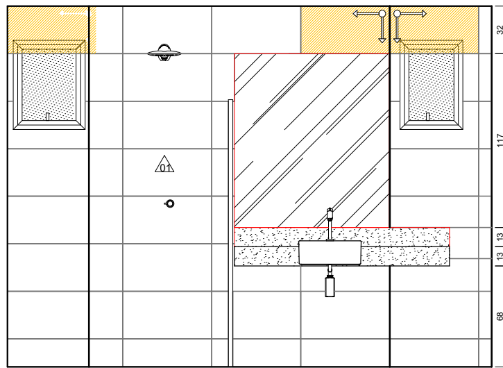
VISTA B ESCALA 1/25
