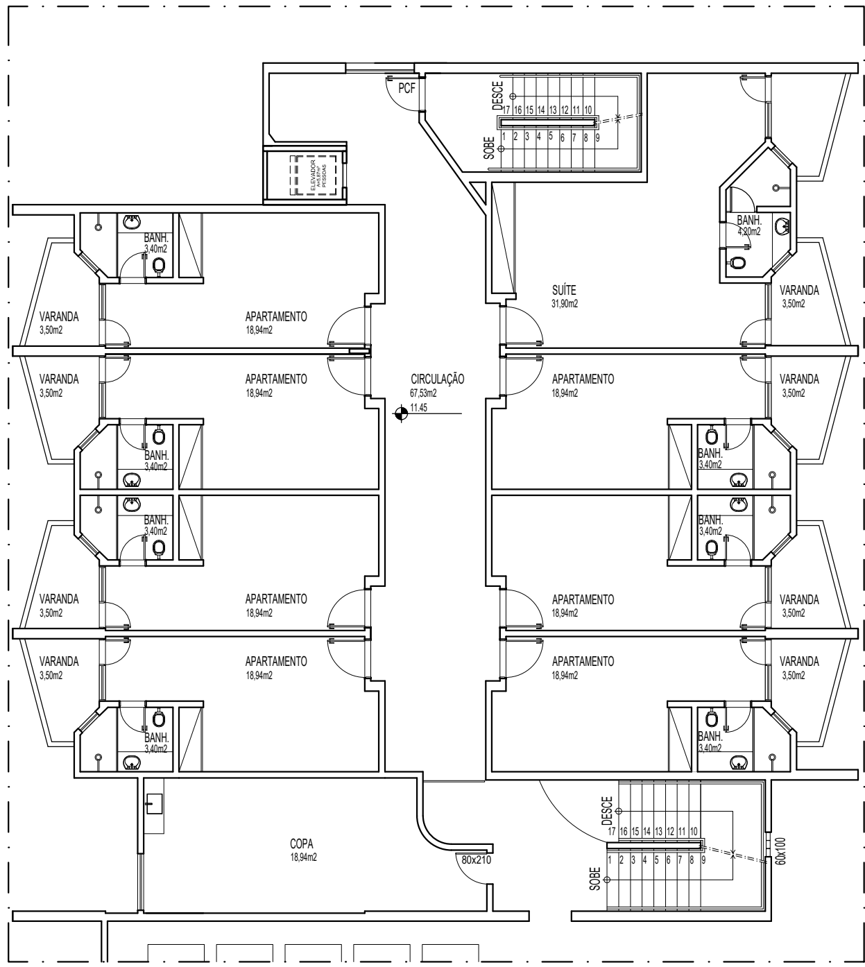
PLANTA BAIXA SUBSOLO EXISTENTE ESCALA 1/125 APTOS 344 A 351
