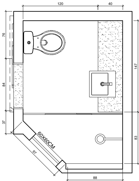
PLANTA BAIXA ESCALA 1/25
