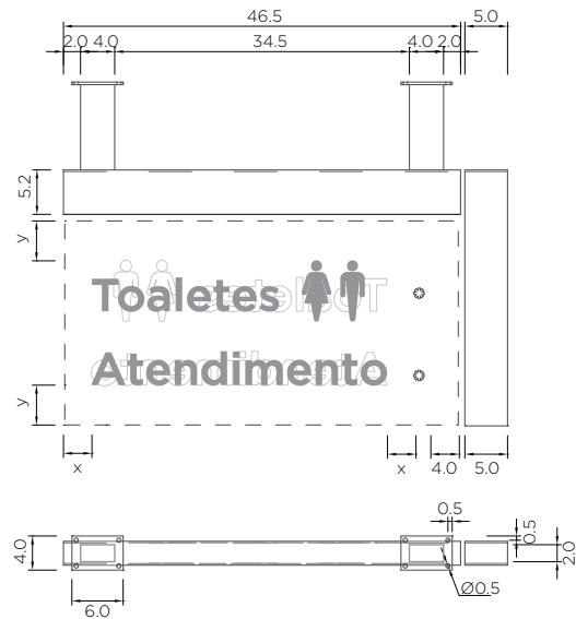
Chapa metálica e textos vistas ortográficas
