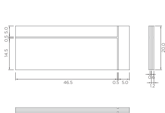
PVC ou MDF vistas ortográficas
