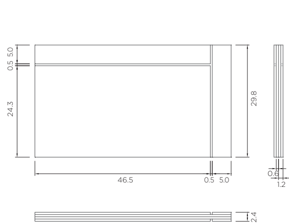
PVC ou MDF vistas ortográficas
