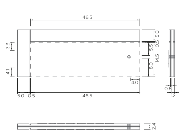
PVC ou MDF vistas ortográficas
