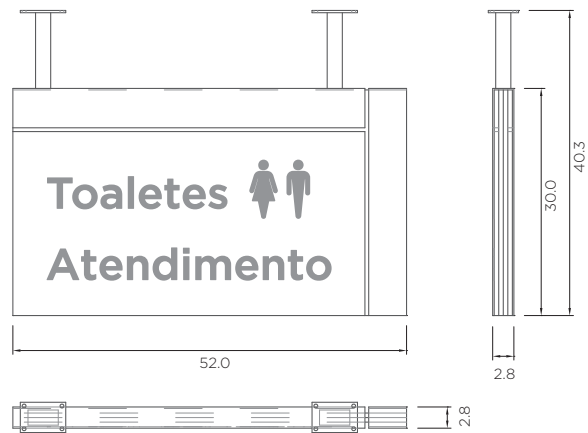
Peças montadas vistas ortográficas
