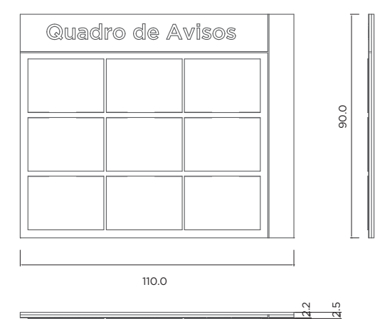
Peças montadas vistas ortográficas
