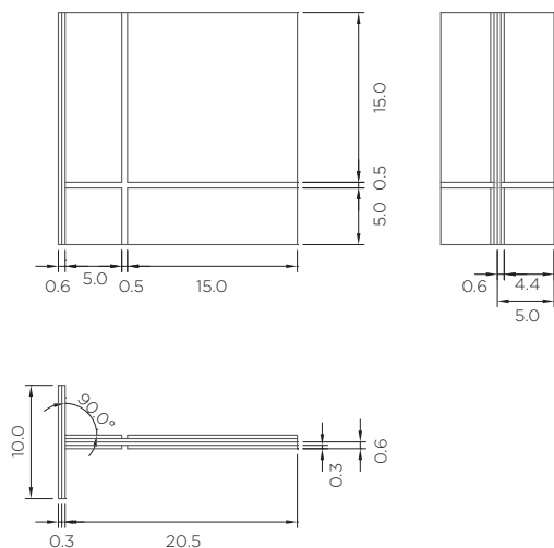
PVC ou MDF vistas ortográficas
