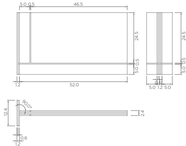
PVC ou MDF vistas ortográficas
