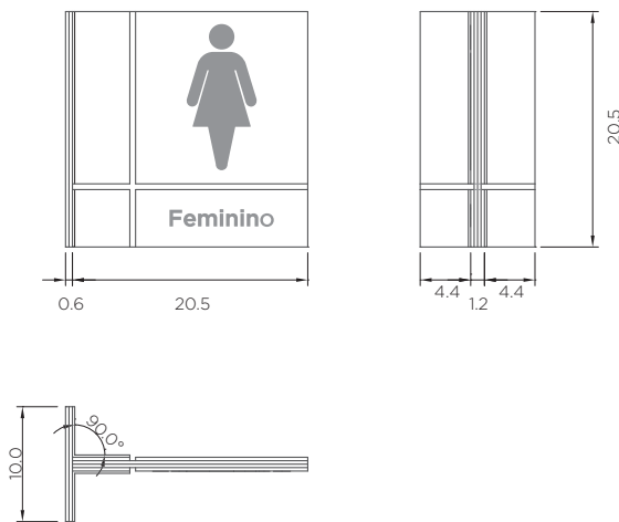
Peças montadas vistas ortográficas
