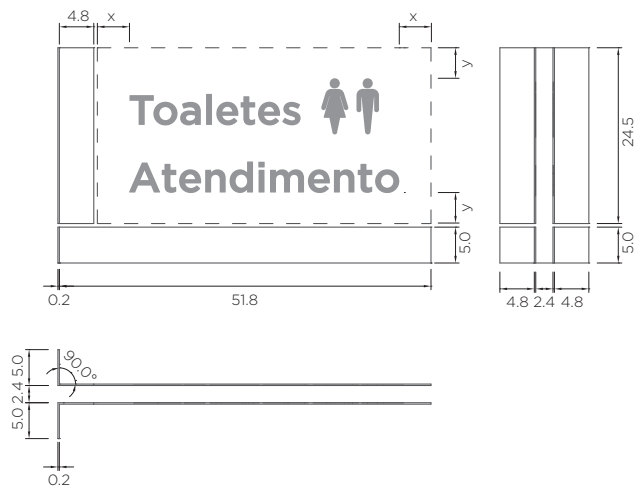
Chapa acrílica e textos vistas ortográficas
