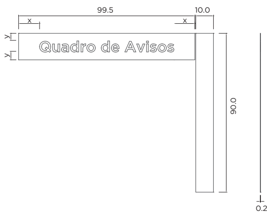
Chapa acrílica e textos vistas ortográficas
