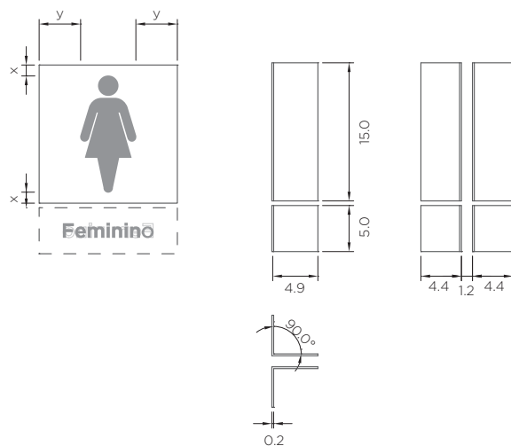
Chapa acrílica e textos vistas ortográficas
