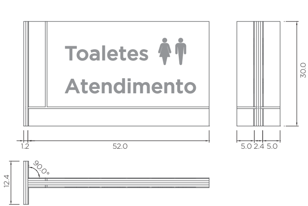
Peças montadas vistas ortográficas
