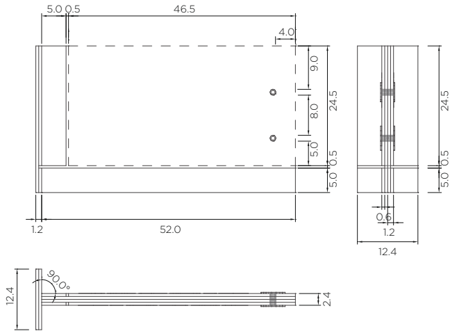
PVC ou MDF vistas ortográficas
