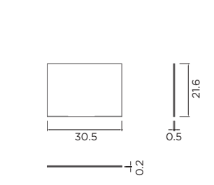
Acrílico cristal vistas ortográficas
