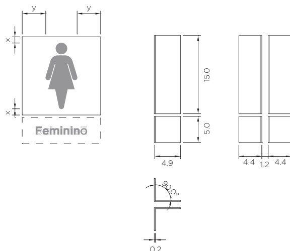
Chapa acrílica e textos vistas ortográficas
