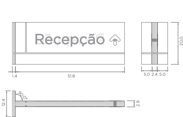
Peças montadas vistas ortográficas
