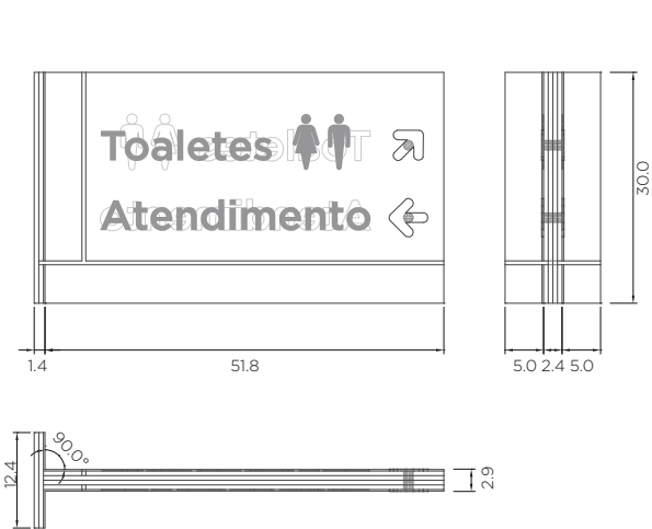
Peças montadas vistas ortográficas
