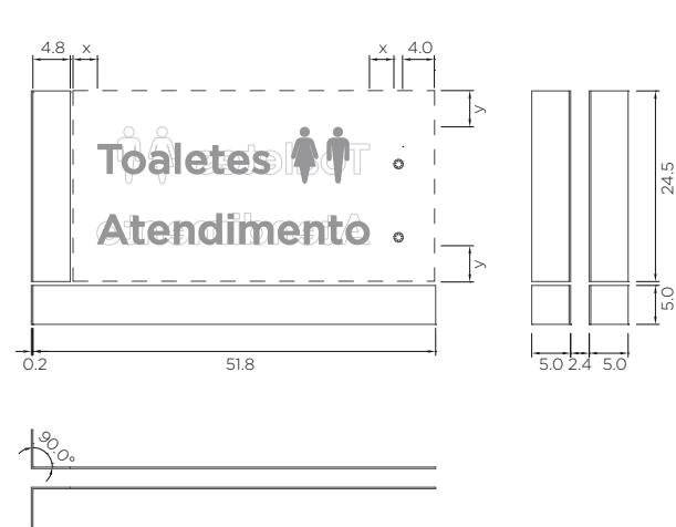
Chapa acrílica e textos vistas ortográficas
