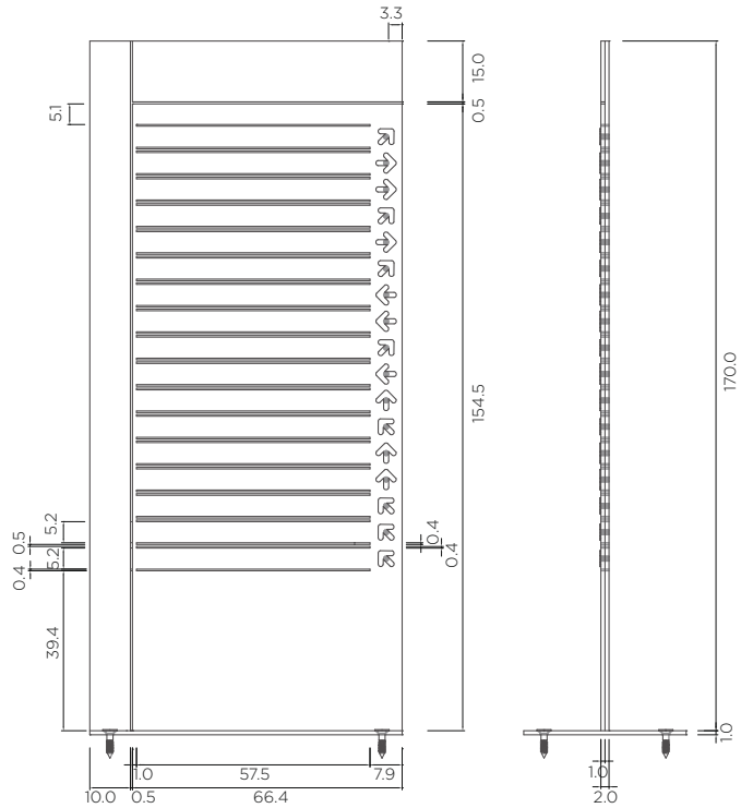
PVC ou MDF vistas ortográficas
