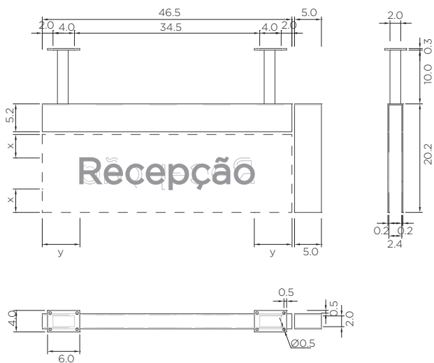
Chapa metálica e textos vistas ortográficas
