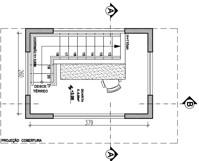
1º PAVIMENTO ESCALA 1/25
