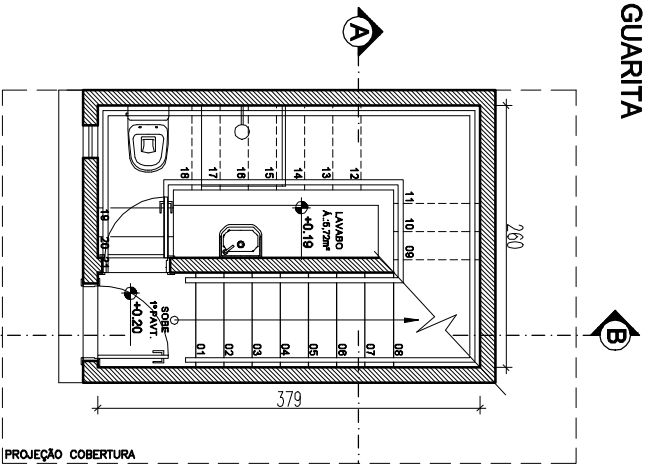
PAVIMENTO TÉRREO ESCALA 1/25
