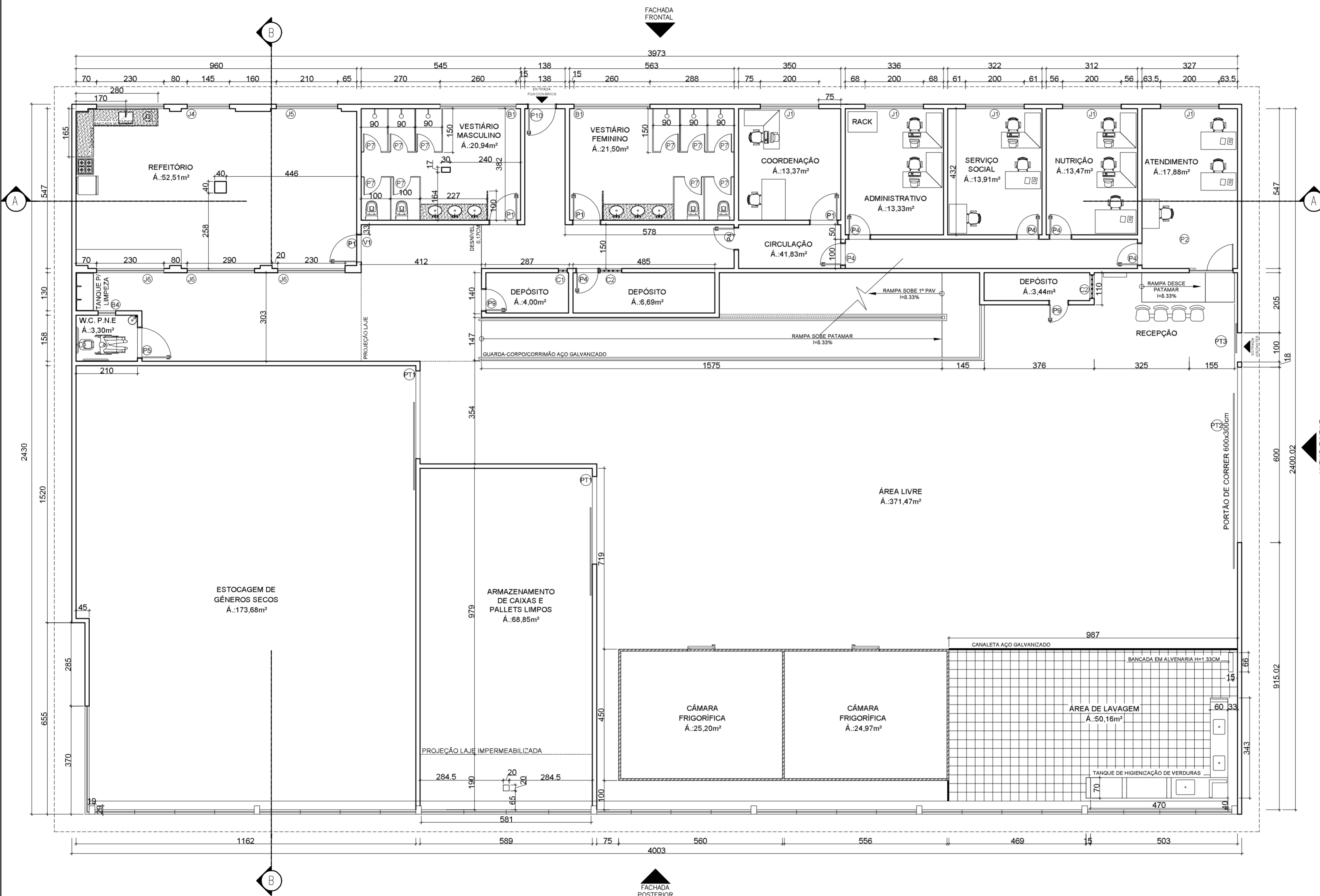
PLANTA BAIXA TÉRREO - GALPÃO ESCALA 1/100
